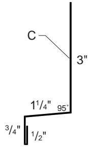
BASE TRIM 170DC-2 without Hat Channel
