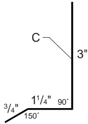
BASE TRIM 170DC-2 without Hat Channel
